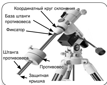
Рис. 6а: Монтровка, штанга противовеса и противовес в сборе (EXOS-2)
