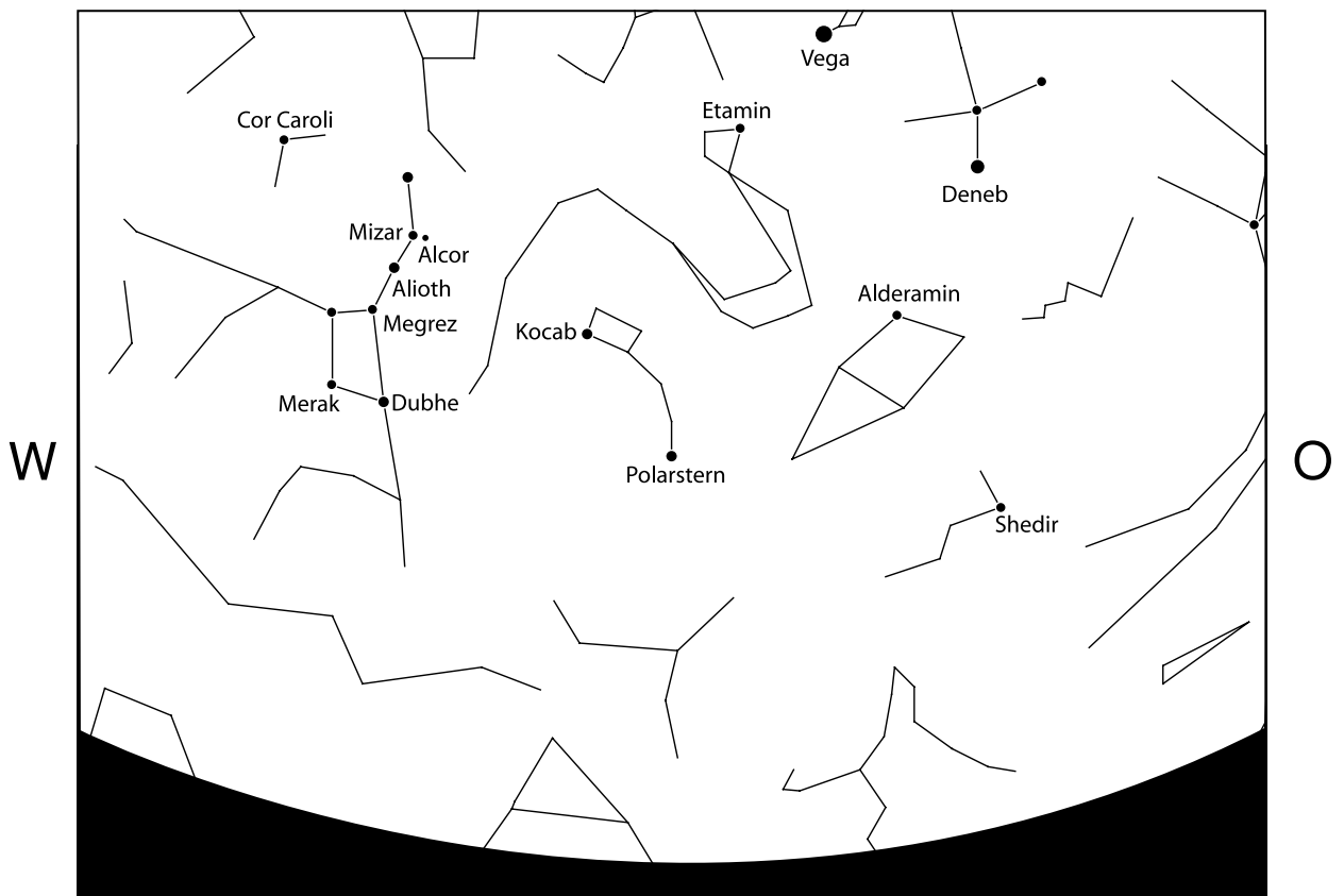
Рис. 52а: Северное полушарие (начало июля, около 22 часов)
