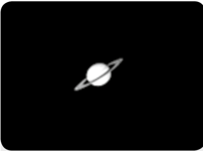
Рис. 44: Сатурн с его системой колец.
