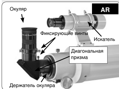
Рис. 10б: Вставьте окуляр в диагональную призму и затяните фиксирующие винты
