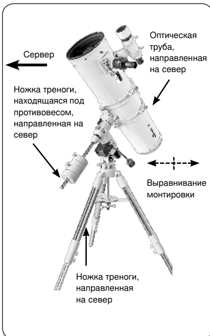
Рис. 16а: Полярное положение, вид сбоку
