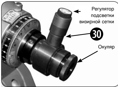
Рис. 35: Полярный искатель*
