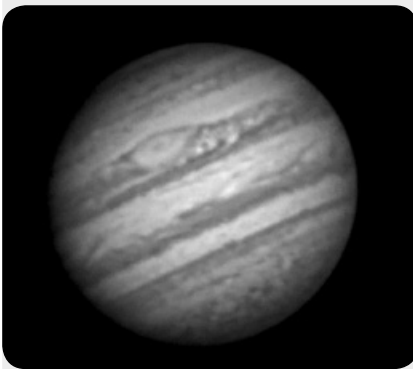
Рис. 43а: Юпитер на большом увеличении. Обратите внимание на детальную структуру облаков.
