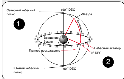
Рис. 33: Небесная сфера
