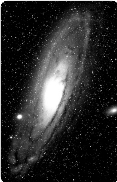
Рис. 47: Галактика Андромеды (M31) – ближайшая к нам спиральная галактика.
