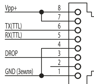
Разъем для подключения к монтировке
