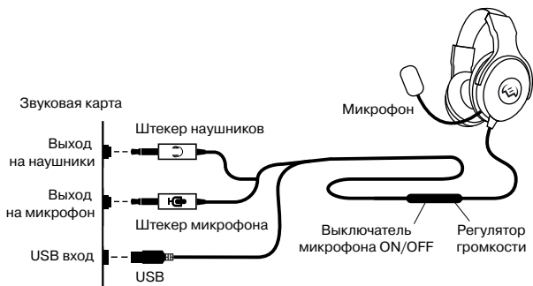
Рис. 4. Схема подключения
